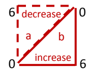
Disduonity Module
