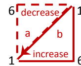
Duonity Module
